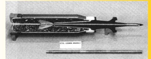
Pénétrateur à l'UA centré en longueur d'un projectile avec sabot.
